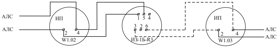
Схема подключения извещателя к АЛС
